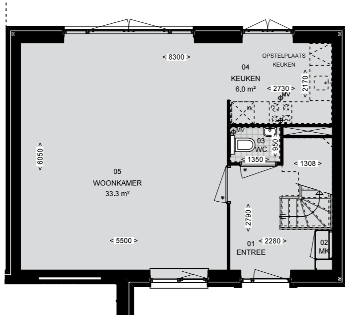
BEGANE GROND Type E1
