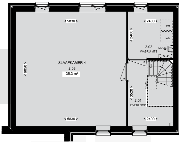
2e VERDIEPING Type E1
