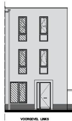
VOORGEVEL LINKS
