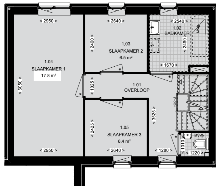
1e VERDIEPING Type E1
