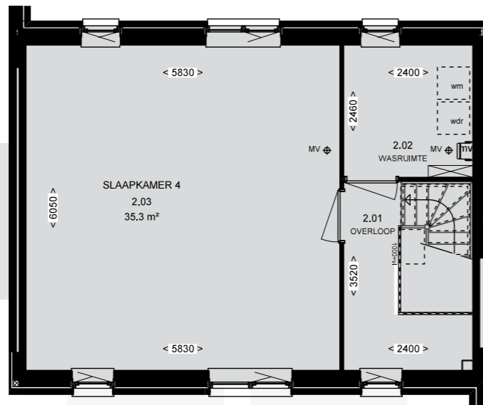
2e VERDIEPING Type E2
