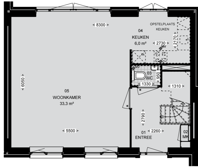
BEGANE GROND Type E2
