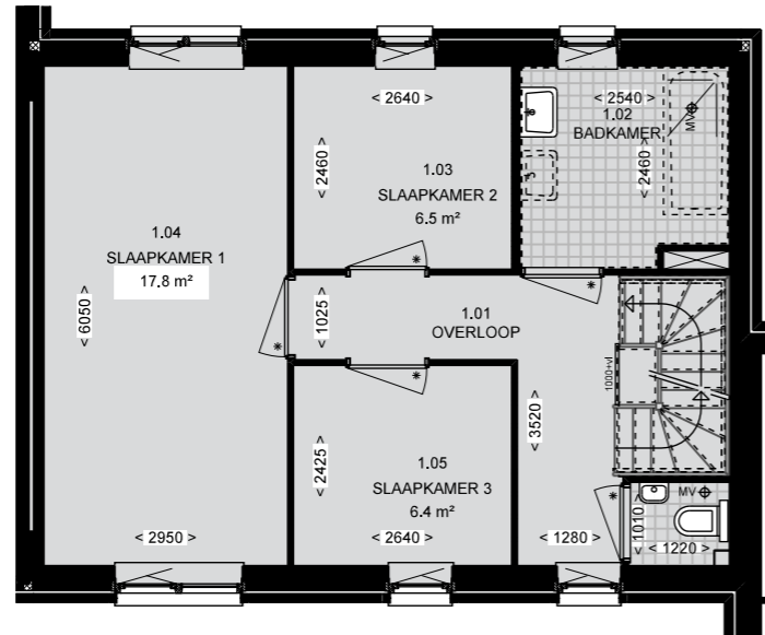
1e VERDIEPING Type E2
